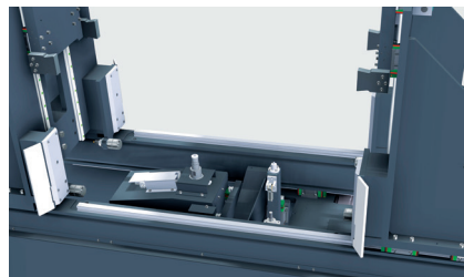
Unité de marquage - fraisage 4 ème axe Milling and marking unit on 4th-face 4-seitiges Fräsen und Markierenheit
